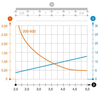
Diagramă încărcare pod de cabluri tip LG 110 VS
