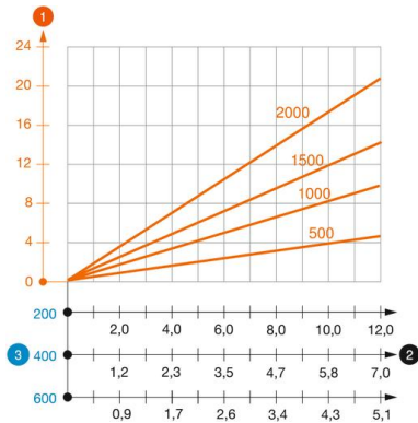
Diagramă încărcare stâlp I tip IS 8 K
