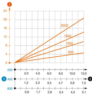
Diagramă încărcare stâlp I tip IS 8 K
